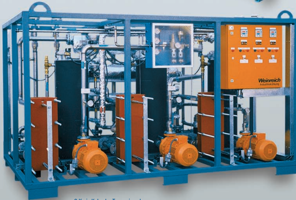
3-Kreis Kalender-Temperieranlage
