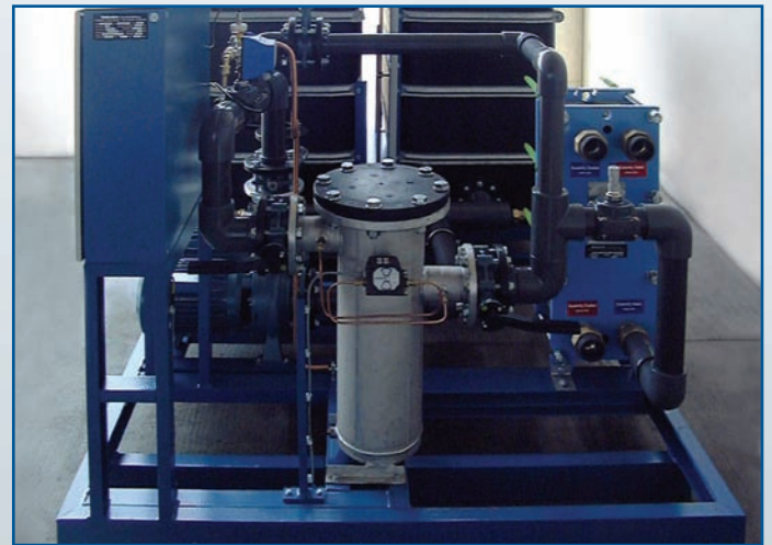
Edelstahl-Feinfilter mit Bypass und Verschmutzungsüberwachung
